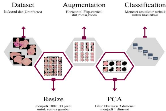
Gambar 4 menunjukkan tahapan model yang diusulkan dalam penelitian ini, step 1 yaitu resize image, step 2 image augmentation, step 3 fitur reduksi dengan PCA, step terakhir classification
