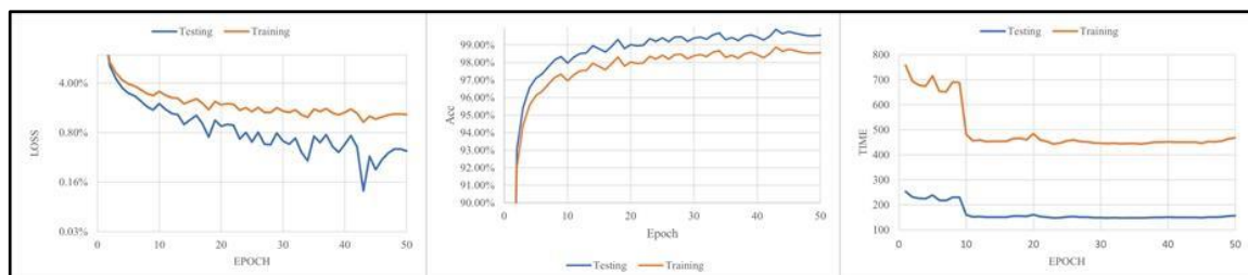
Gambar 10. Grafik Perbandingan loss , akurasi dan waktu komputasi. Gambar sebelah kiri menunjukkan grafik loss , gambar tengah grafik akurasi, dan sebelah kanan grafik waktu komputasi
