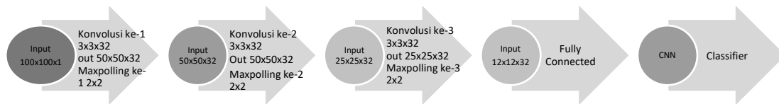
Gambar 6. Arsitektur CNN model yang diusulkan
